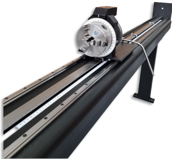
Positioner
